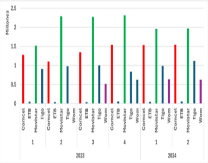
Total de reconexiones móviles por operador – Trimestral
